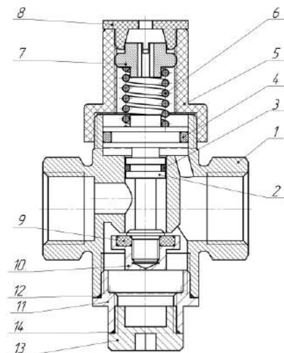
Рисунок 2 – Общий вид и конструкция изделия
